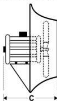
Acoplamiento Directo con cono de succión (AGDC) (Direct drive with inlet cone)
