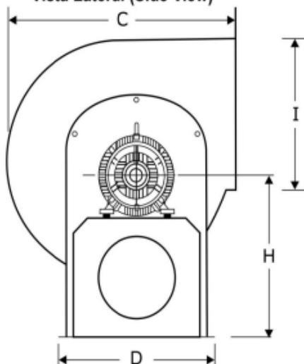
DIMENSIONES GENERALES (DIMENSIONS)
