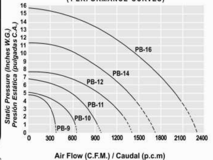
CURVAS DE OPERACIÓN (PERFORMANCE CURVES)
