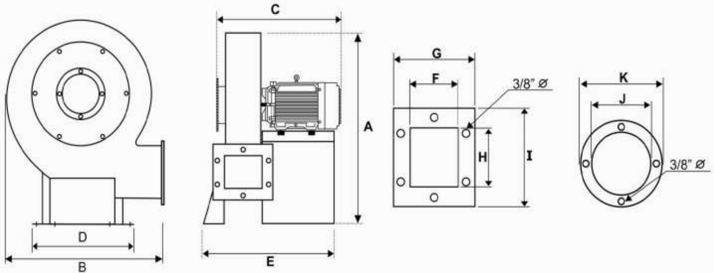
DIMENSIONES GENERALES (DIMENSIONS)
