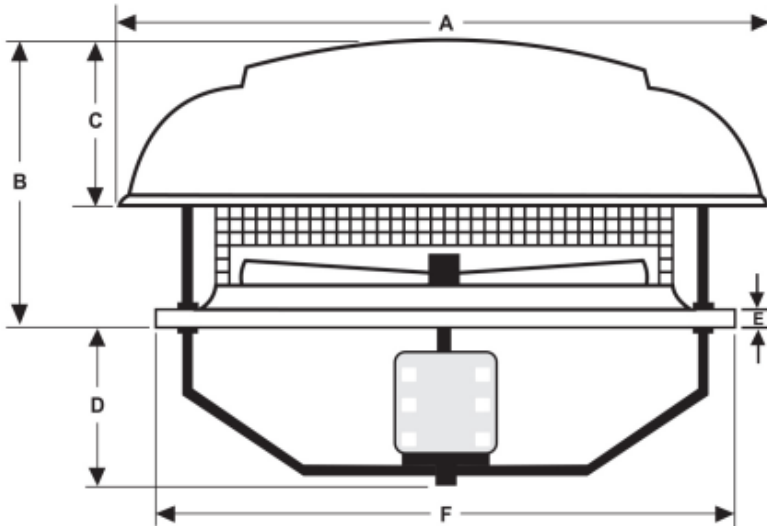
DIMENSIONES GENERALES (DIMENSIONS)
