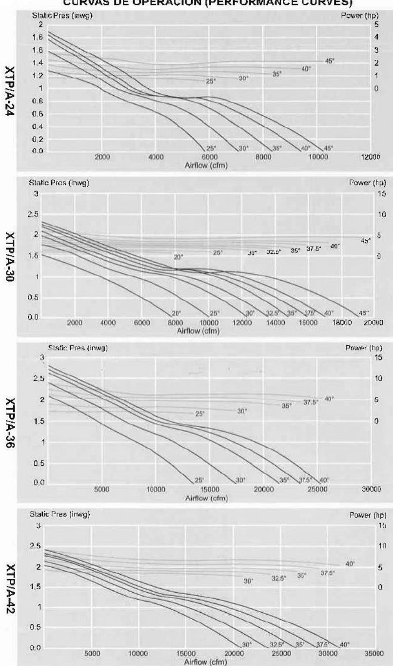
CURVAS DE OPERACIÓN (PERFORMANCE CURVES)
