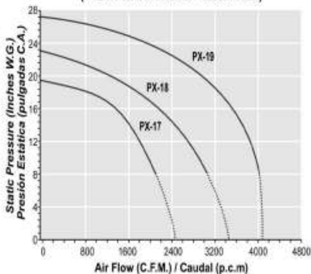
CURVAS DE OPERACIÓN (PERFORMANCE CURVES)
