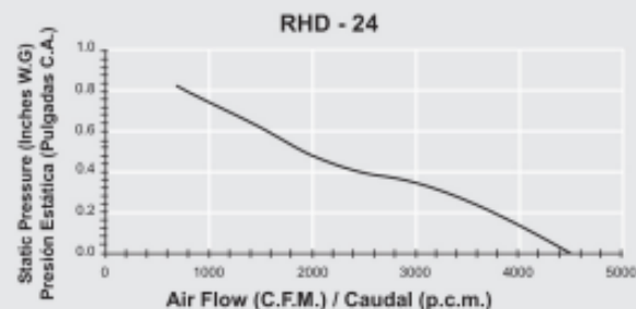
CURVAS DE OPERACIÓN (PERFORMANCE CURVES)
