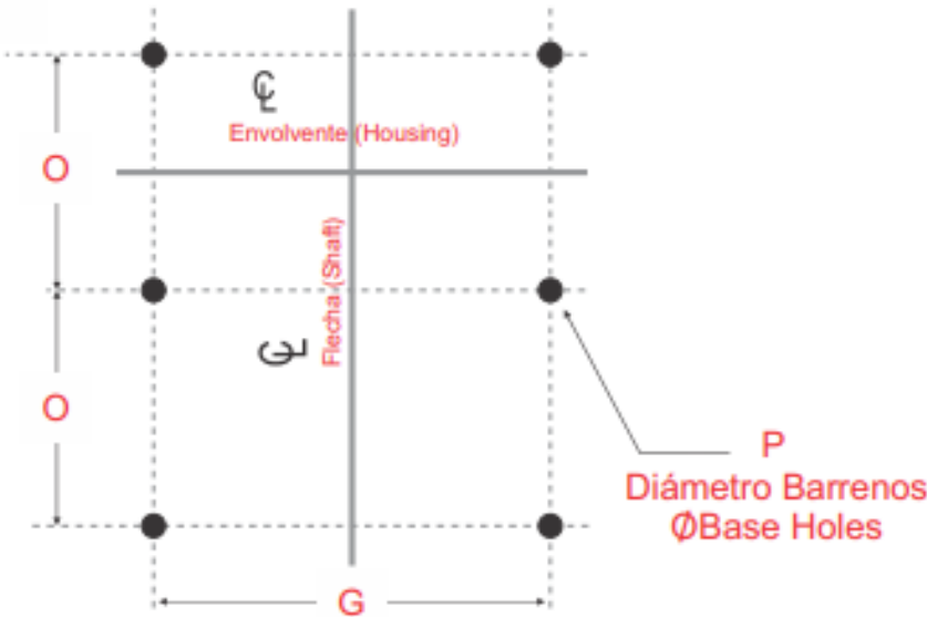
Vista planta para barrenos Foundation plan
