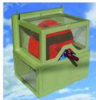
Guarda de protección para el conjunto de la turbina centrífuga-flecha-chumacera (wheel assembly guard)
