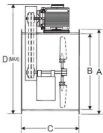
DIMENSIONS
