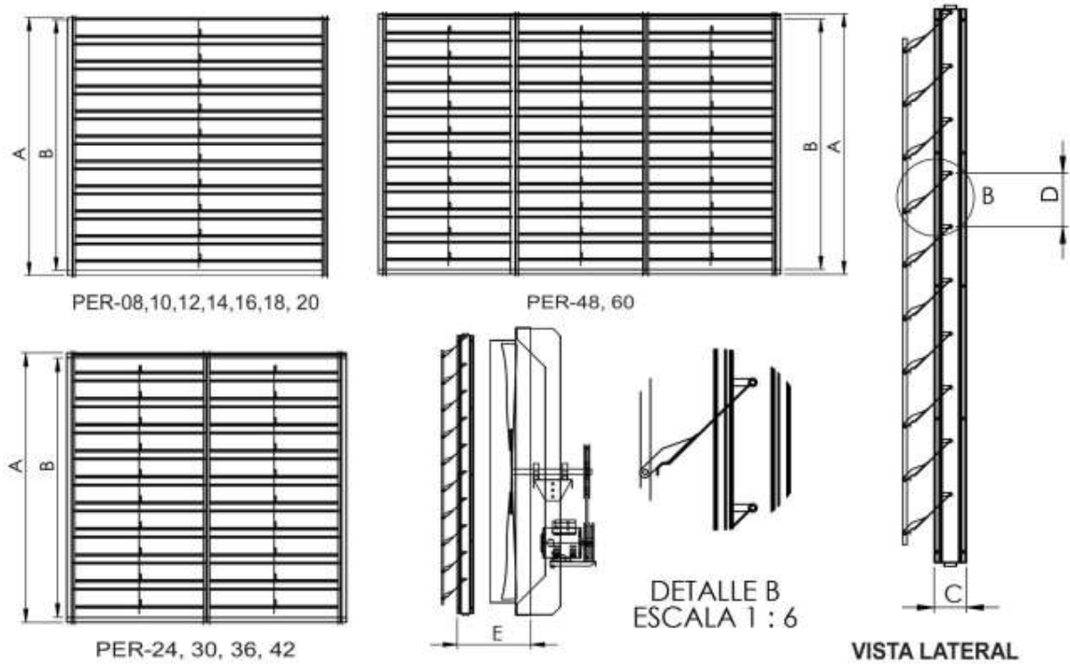
DIMENSIONES GENERALES ( DIMENSIONS )
